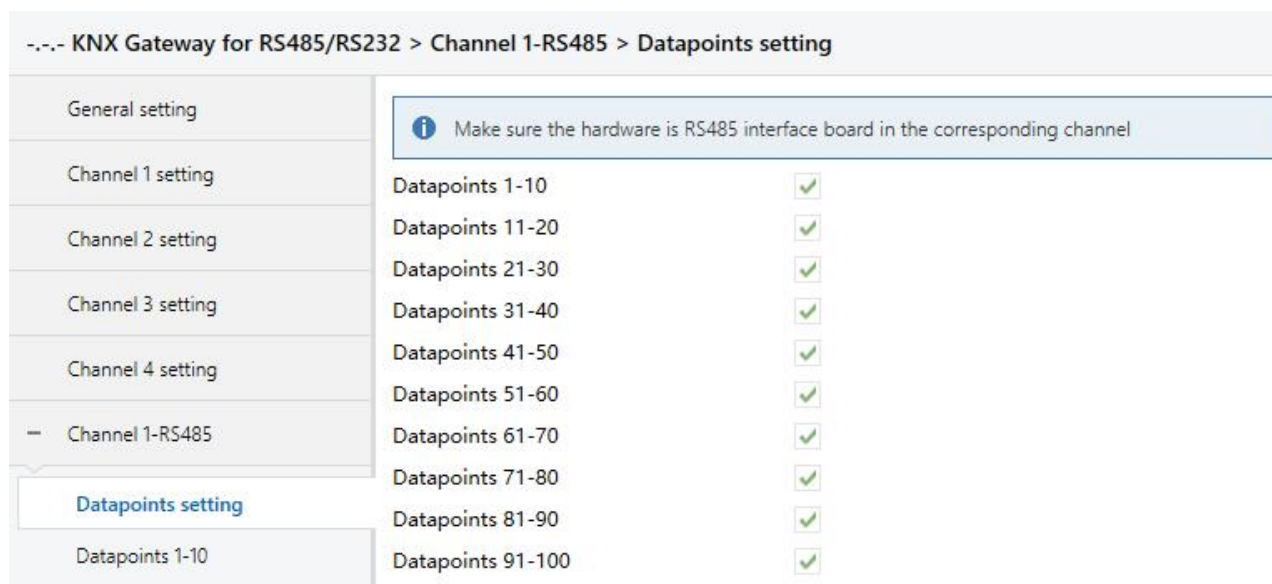
Fig.5.4.1 "Datapoints setting" parameter window
