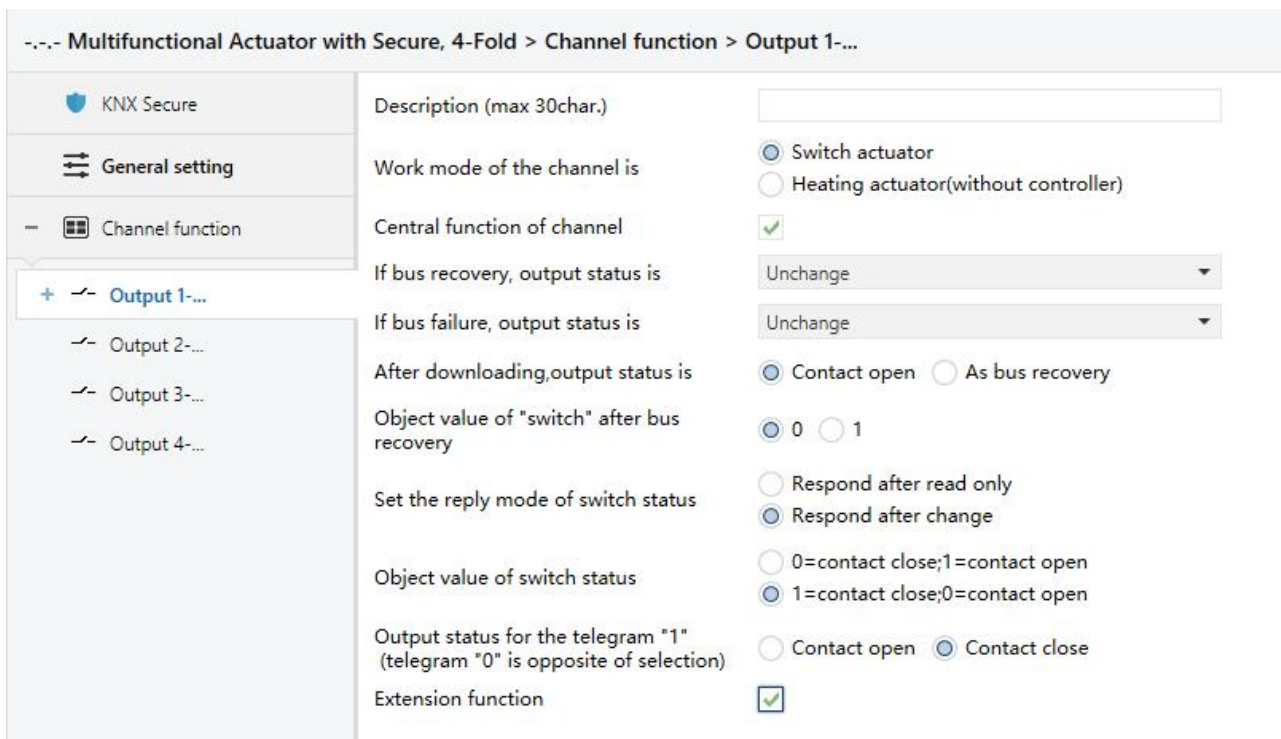
Fig. 4.4.1(1) Parameter window "Output X: Switch actuator"
