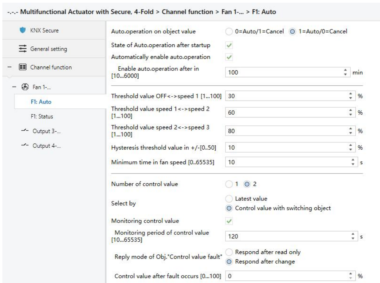
Fig. 4.8.2.1 Parameter window "Fx: Auto."
