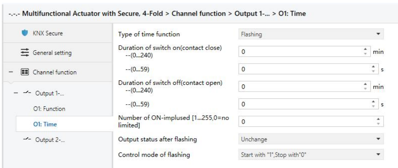
Fig. 4.4.2.2 Parameter window "Ox: Time-Flashing"
