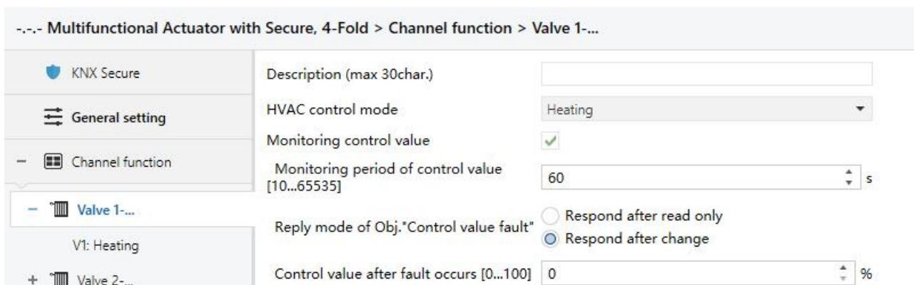
Fig. 4.9(2) Parameter window “Valve X General--Heating”
