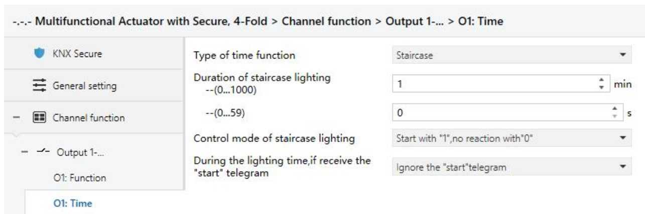
Fig. 4.4.2.3 Parameter window "Ox: Time-Staircase"
