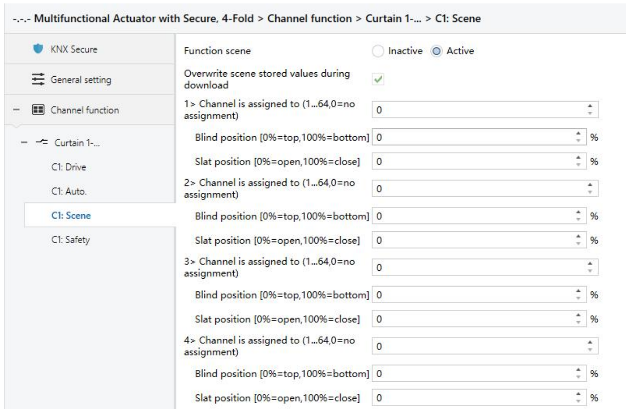
Fig. 4.6.1.3 Parameter window “Cx: Scene”
