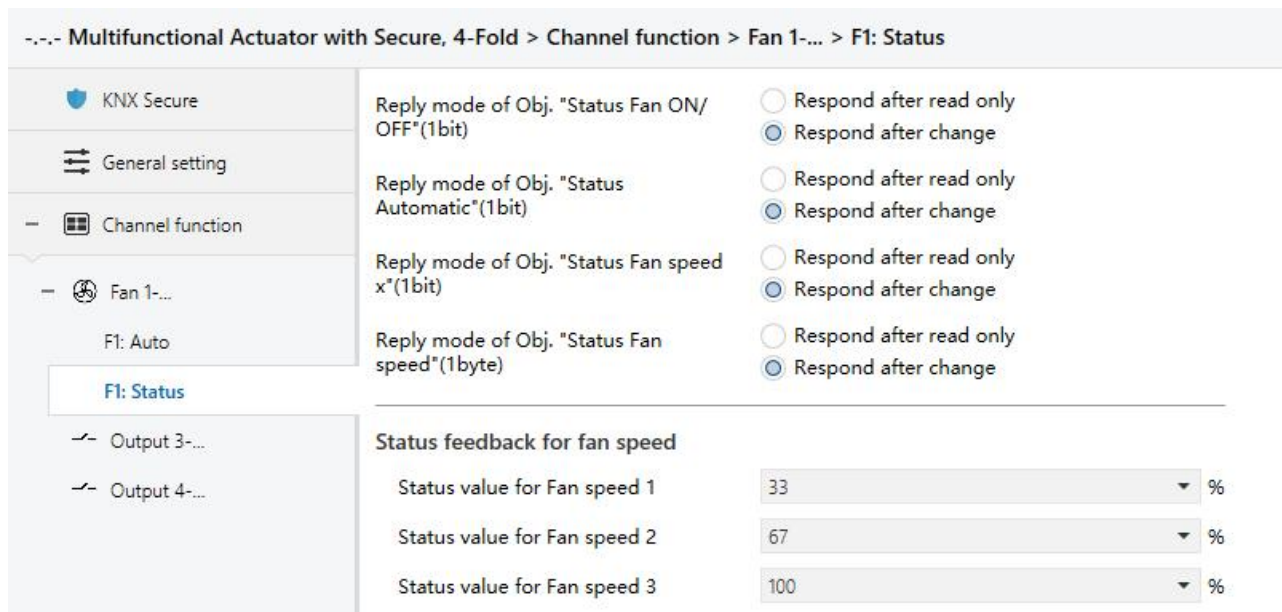
Fig. 4.8.2.2 Parameter window "Fx: Status"
