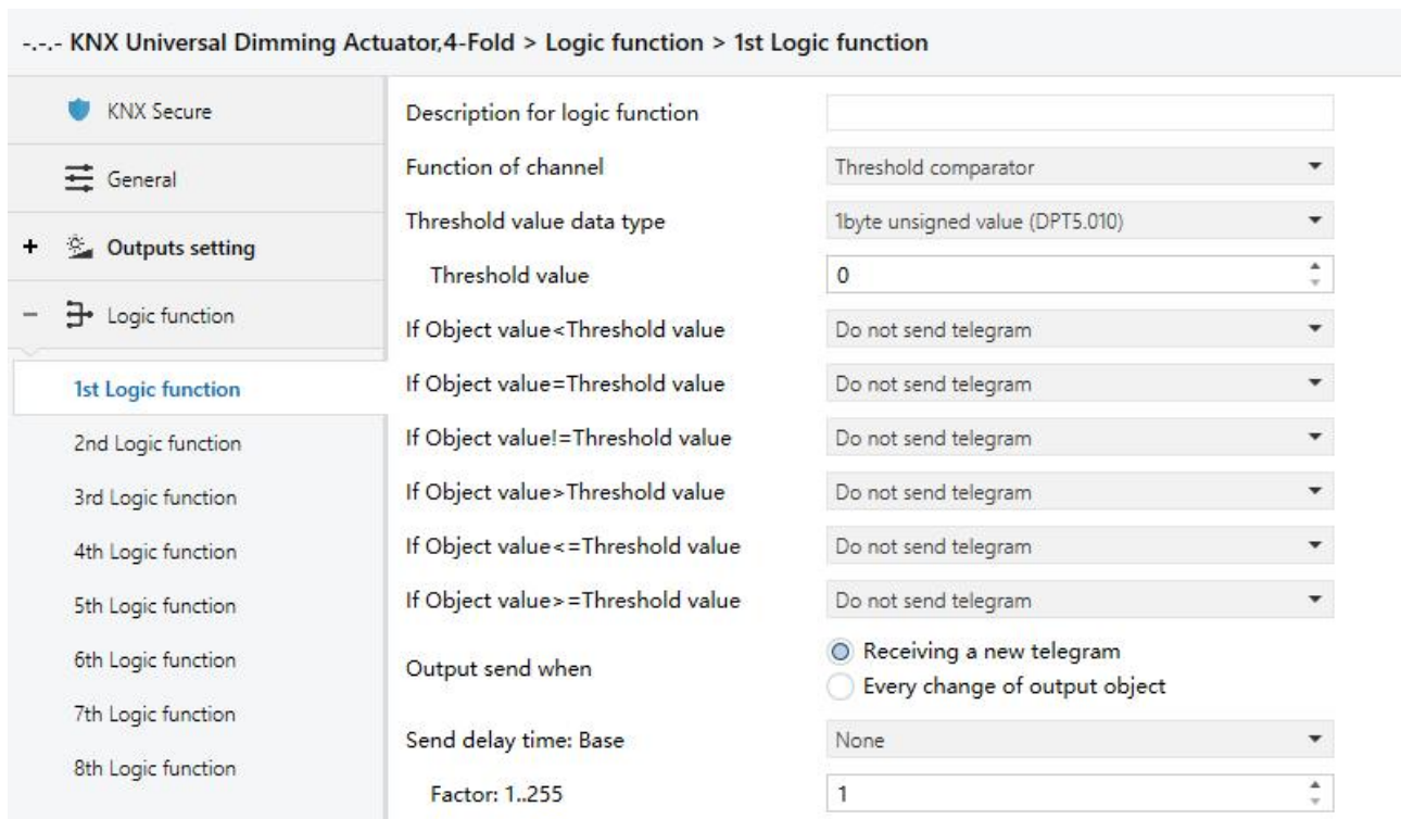
Fig.5.4.3 "Threshold comparator" parameter window
