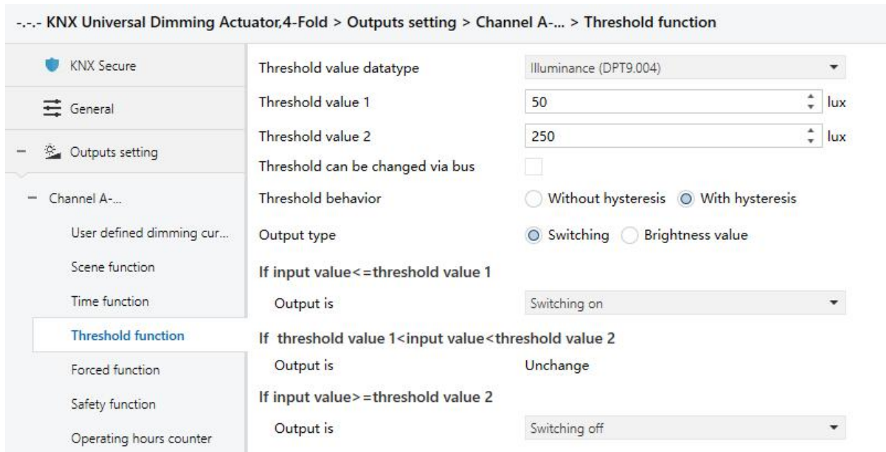
Fig.5.3.3.3 "Threshold function" parameter window
