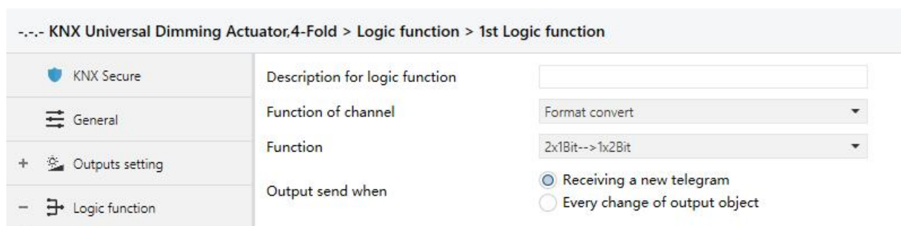
Fig.5.4.4 "Format convert" parameter window
