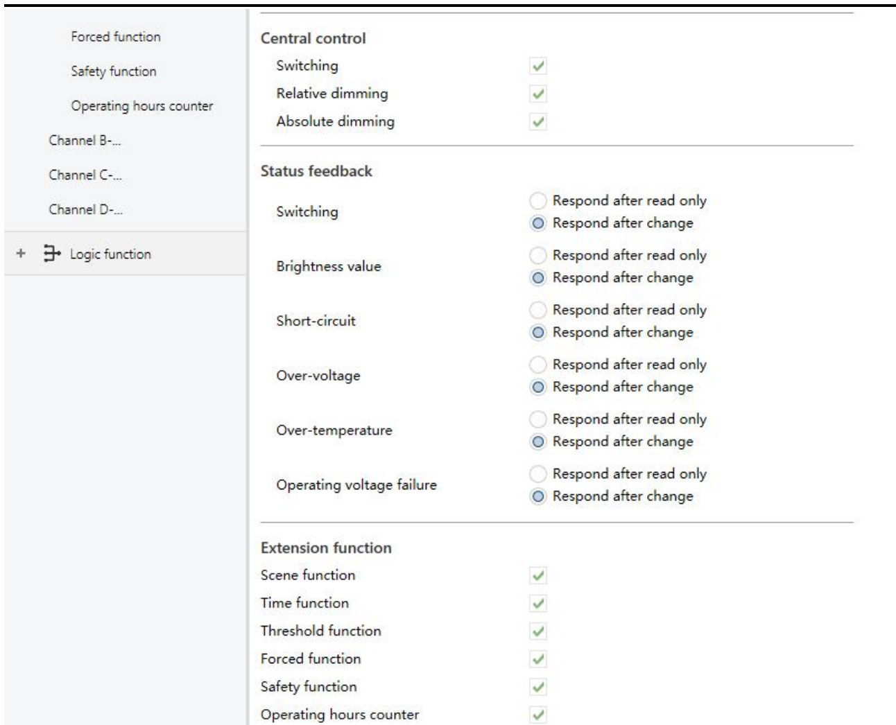
Fig.5.3.1(2) "Channel" parameter window
